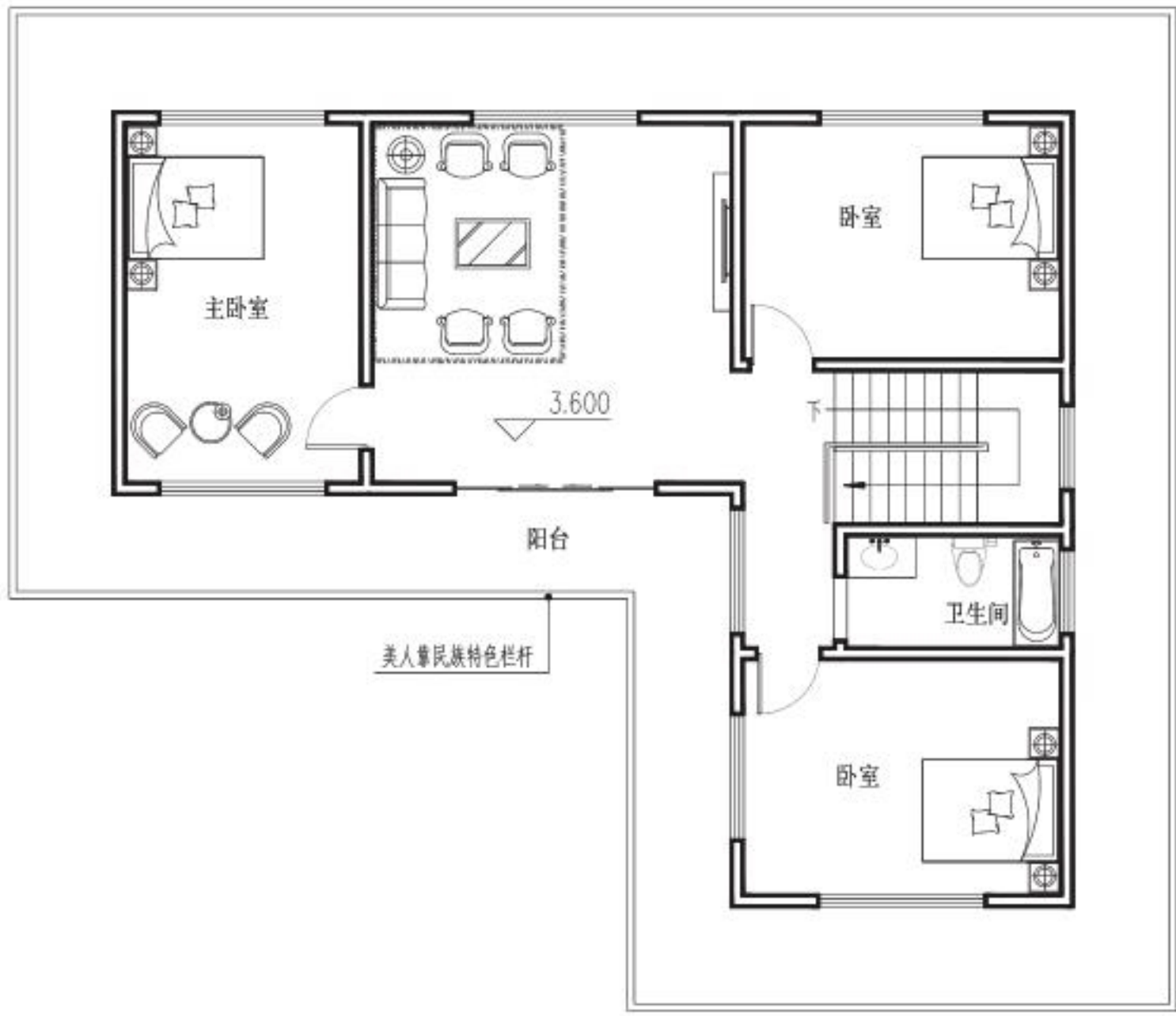
二层平面图
