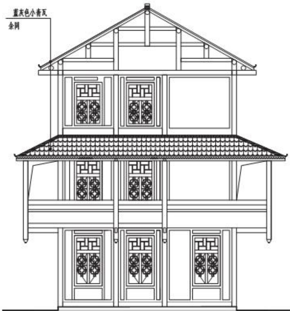
左侧立面图
