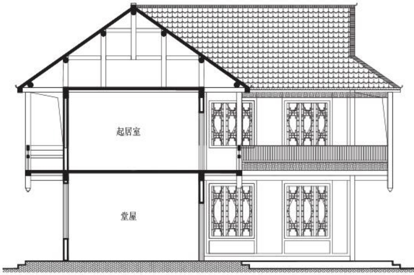
剖面图
