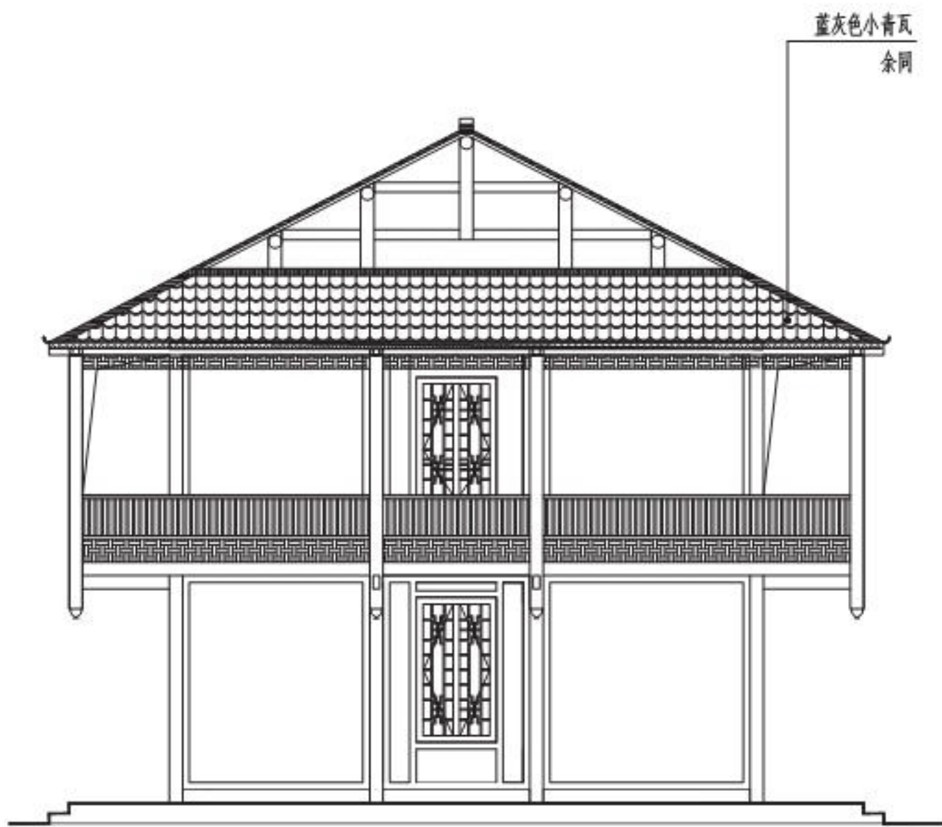
侧立面图
