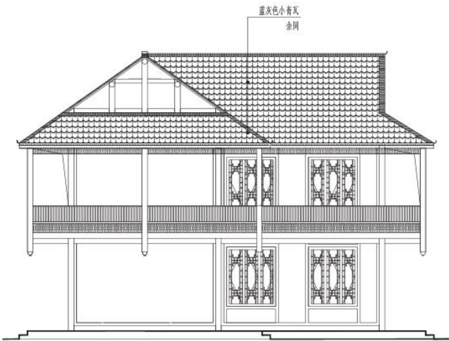
侧立面图
