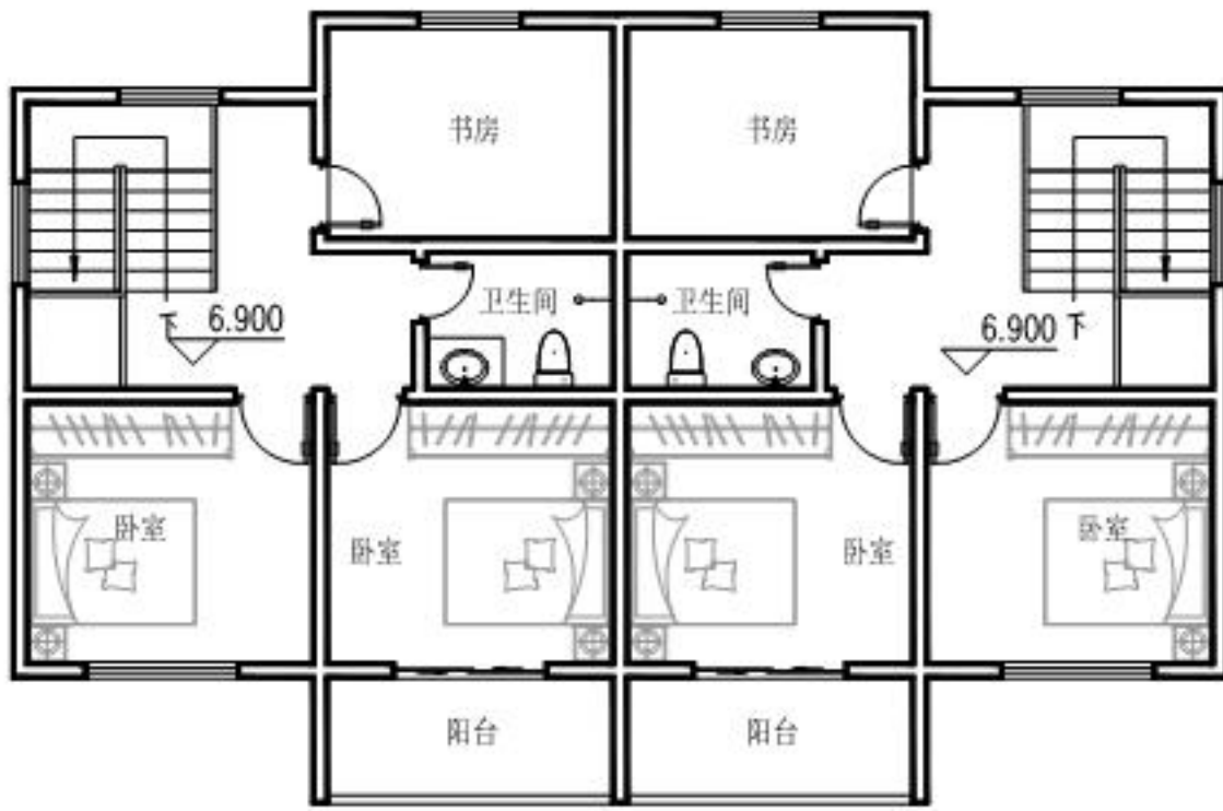
三层平面图
