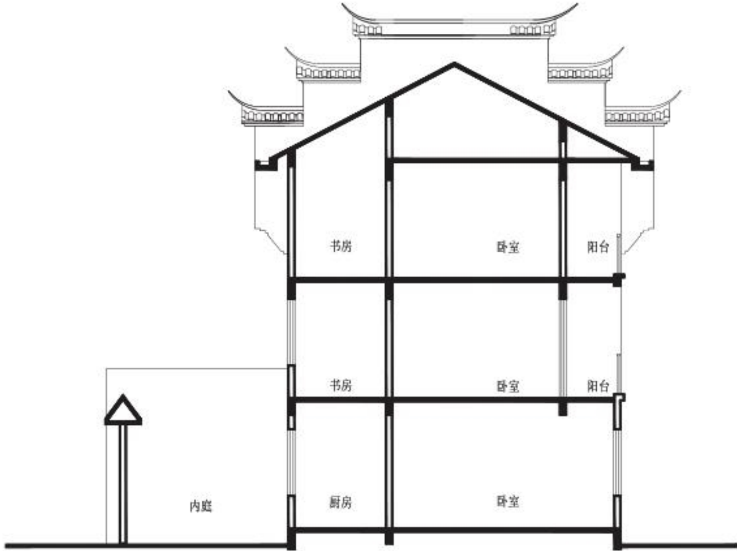
剖面图
