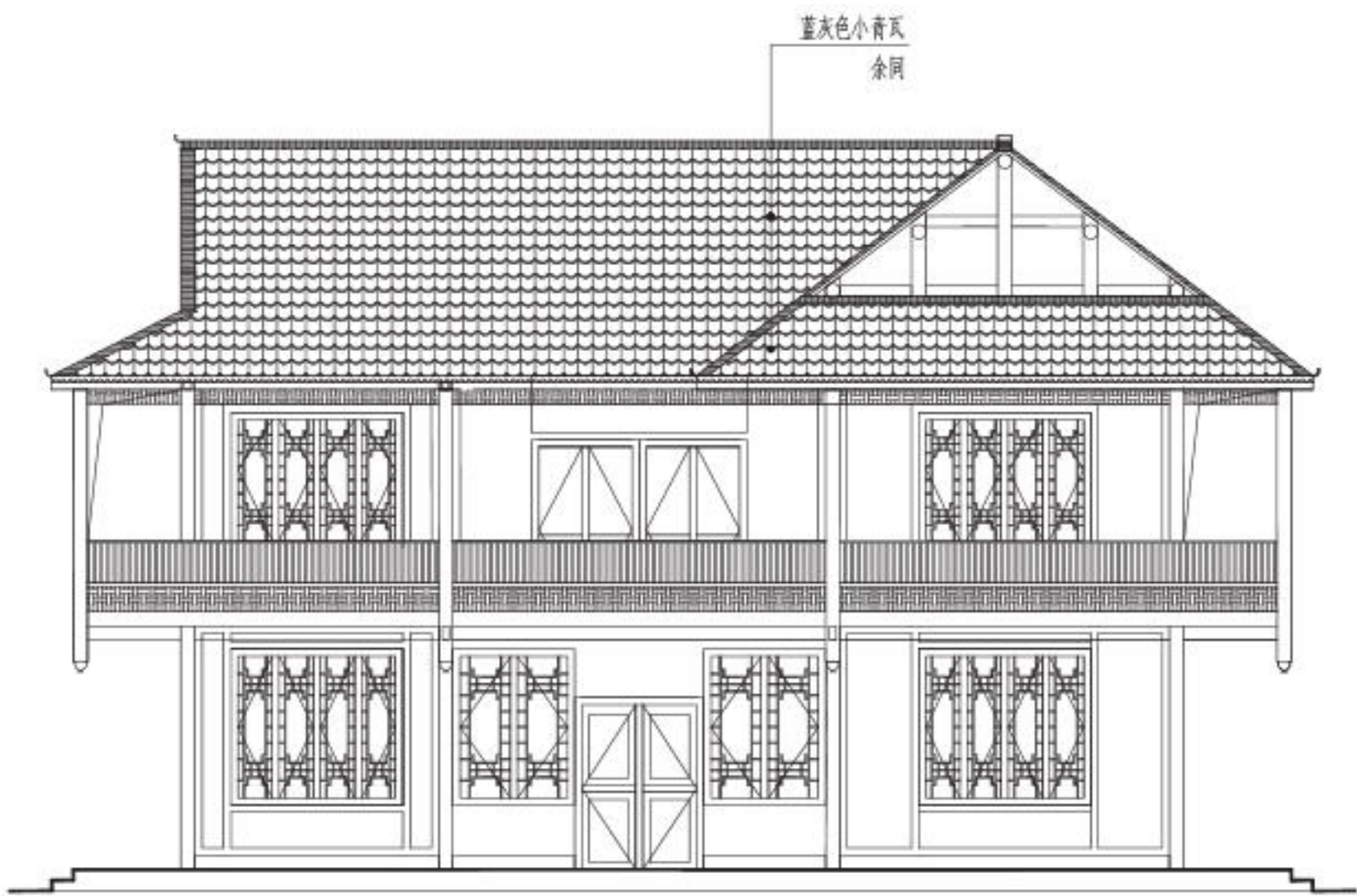
正立面图
