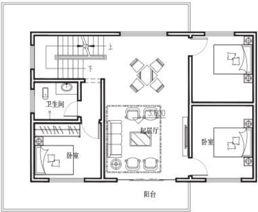
二层平面图
