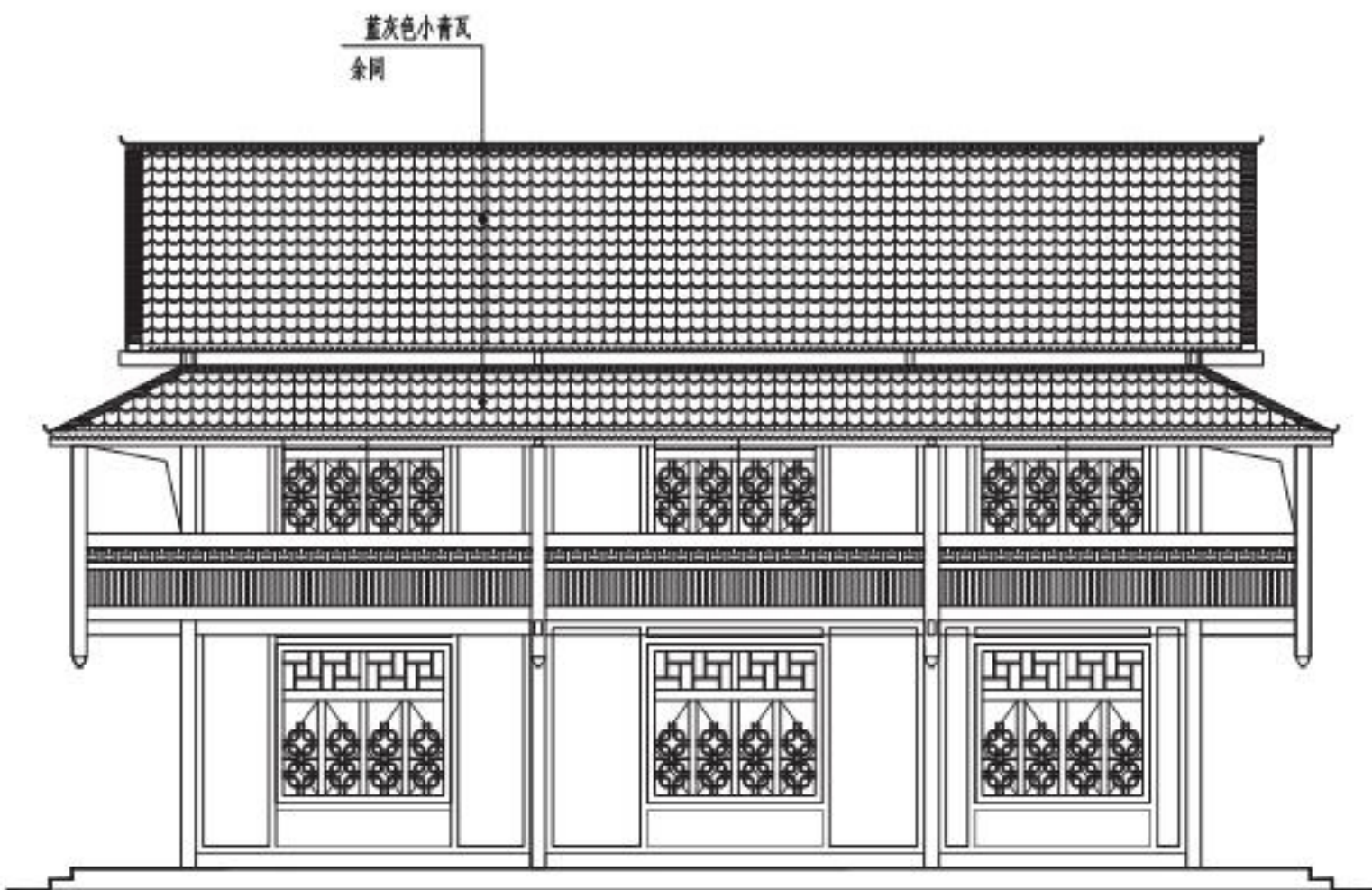
背立面图
