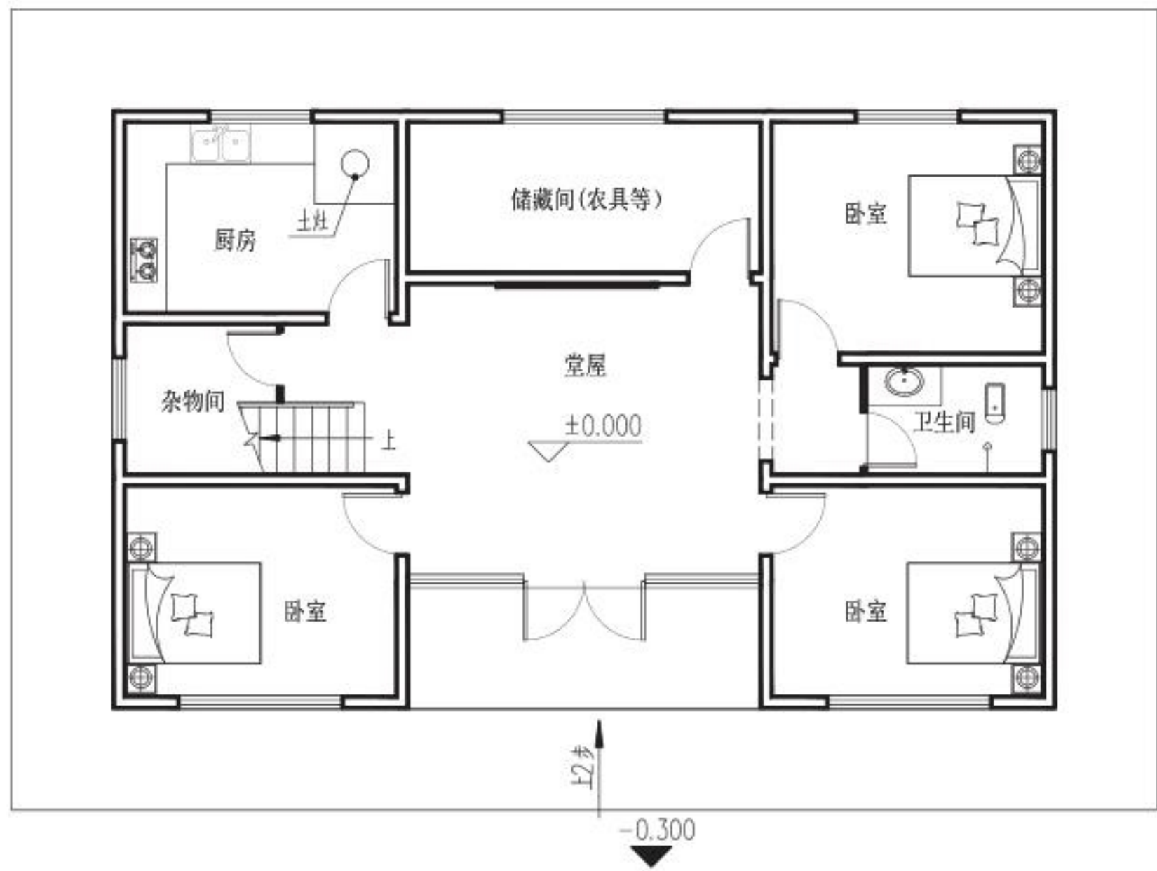
一层平面图
