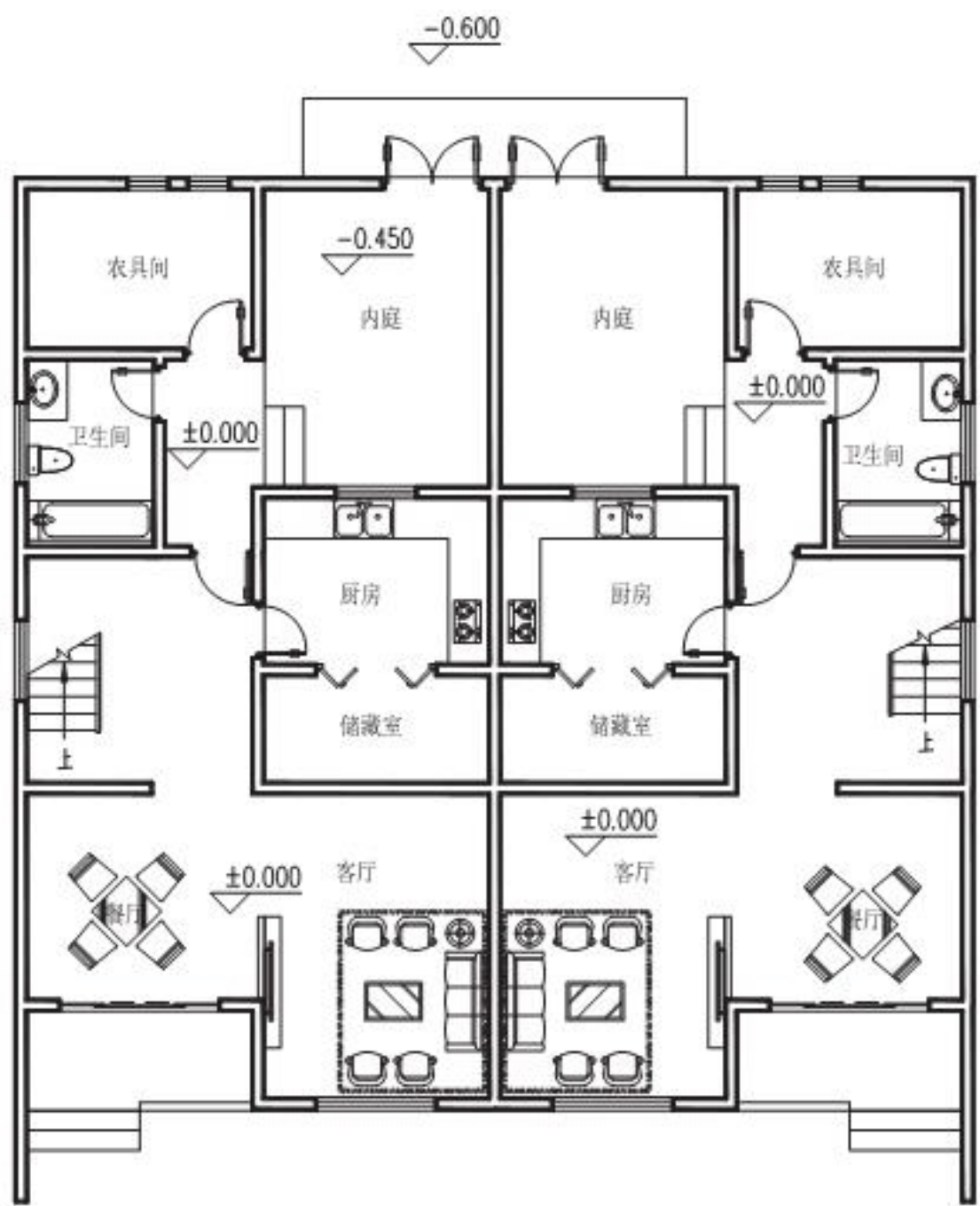
一层平面图
