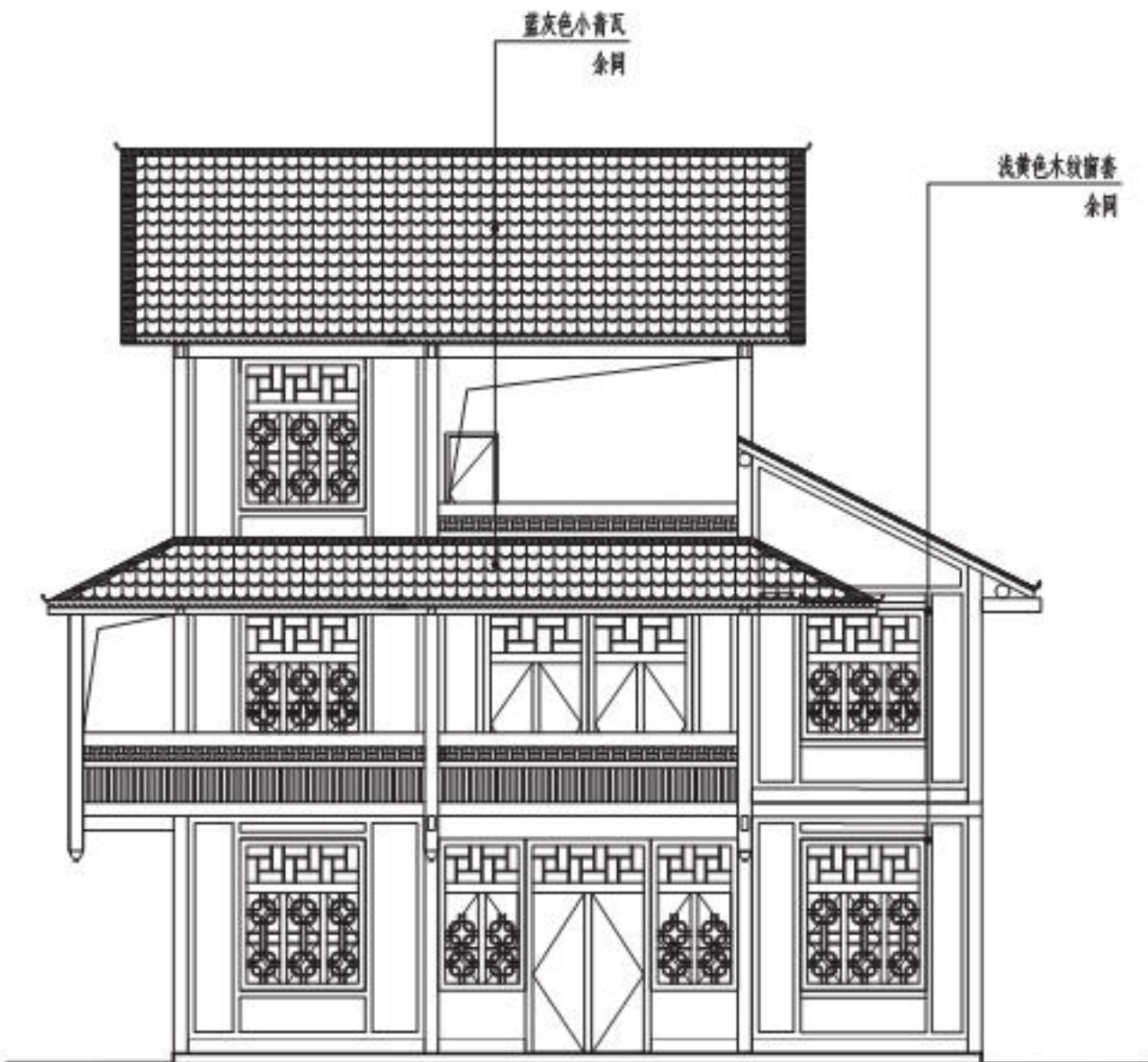
正立面图
