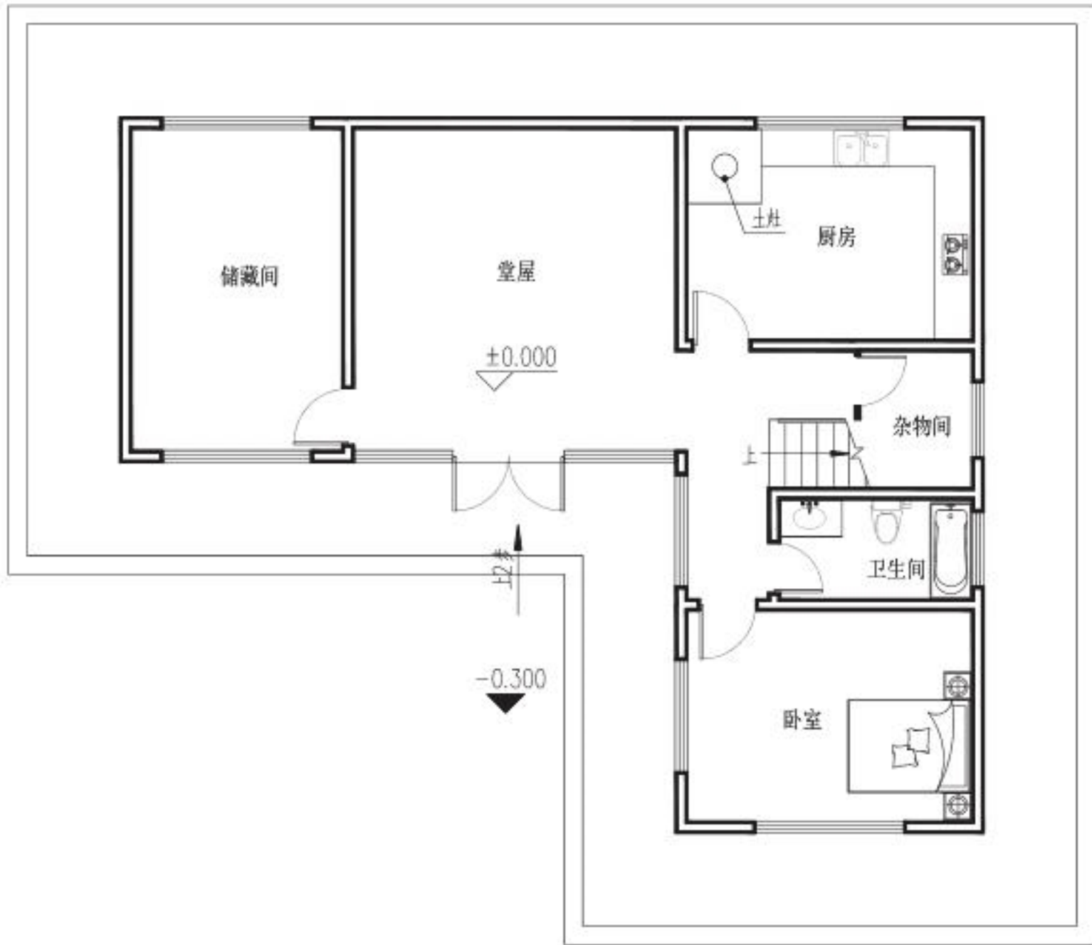
一层平面图
