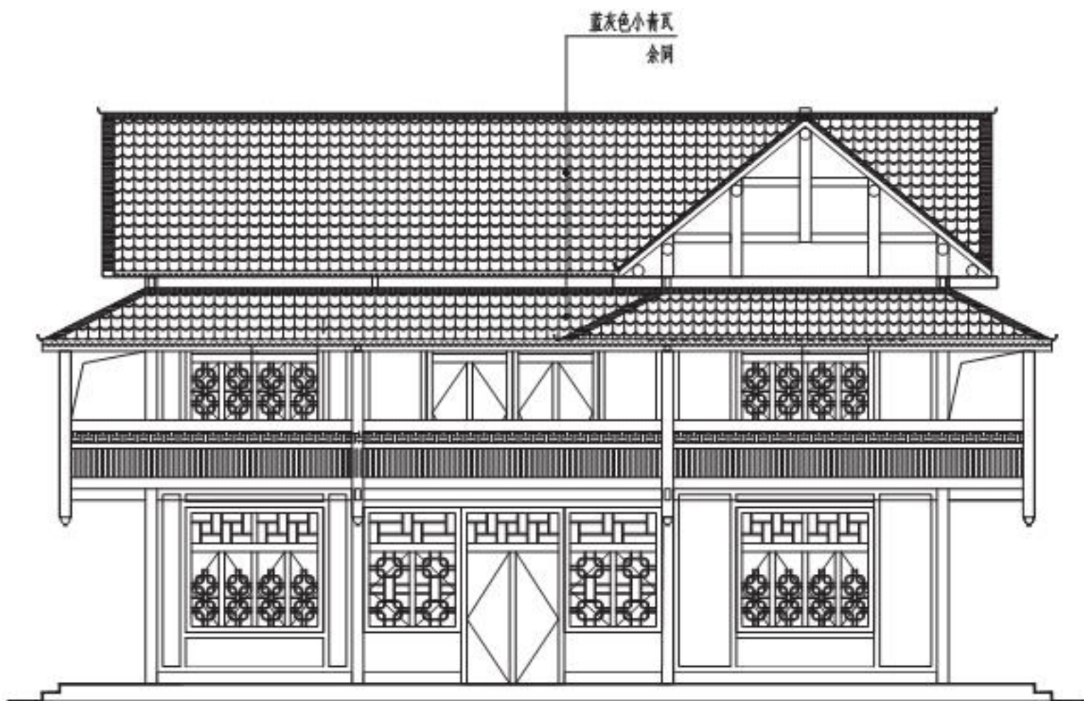
正立面图
