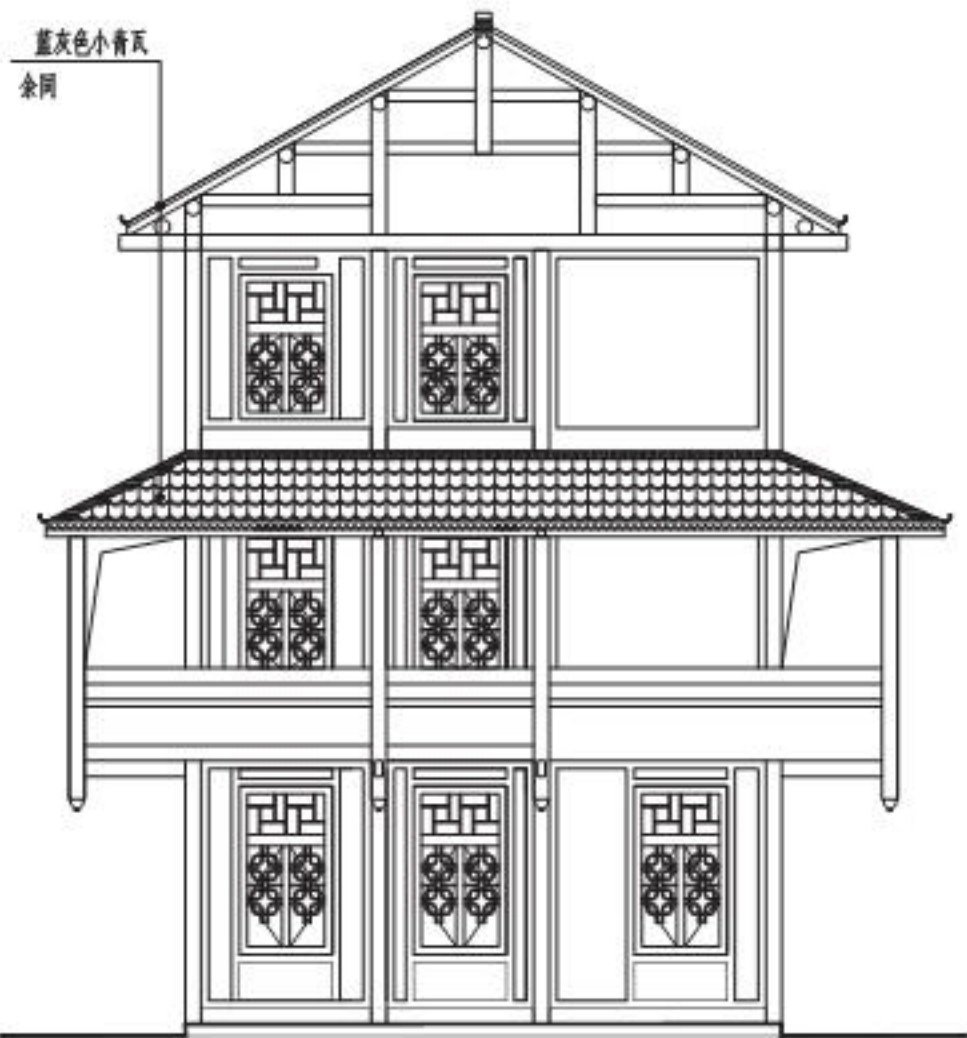
右侧立面图
