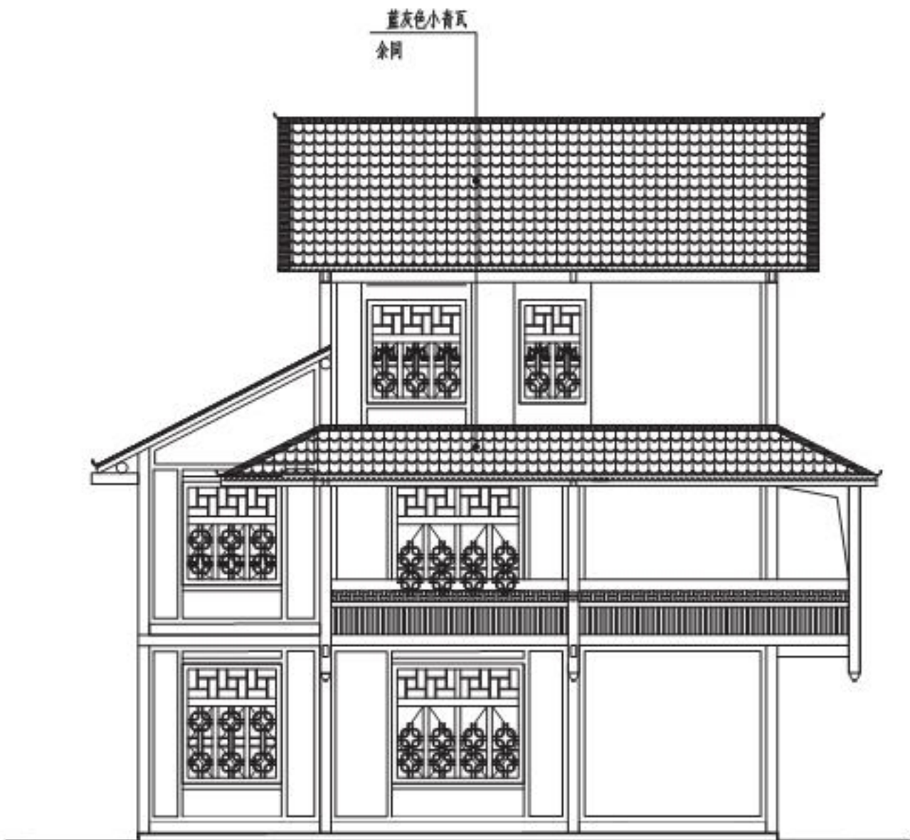
背立面图
