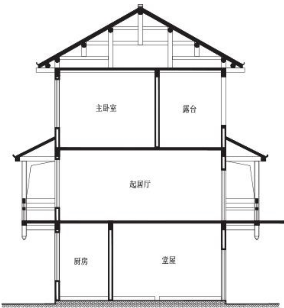
剖面图
