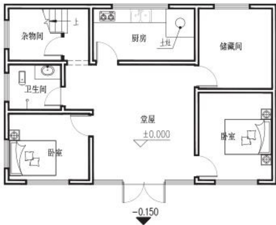
一层平面图
