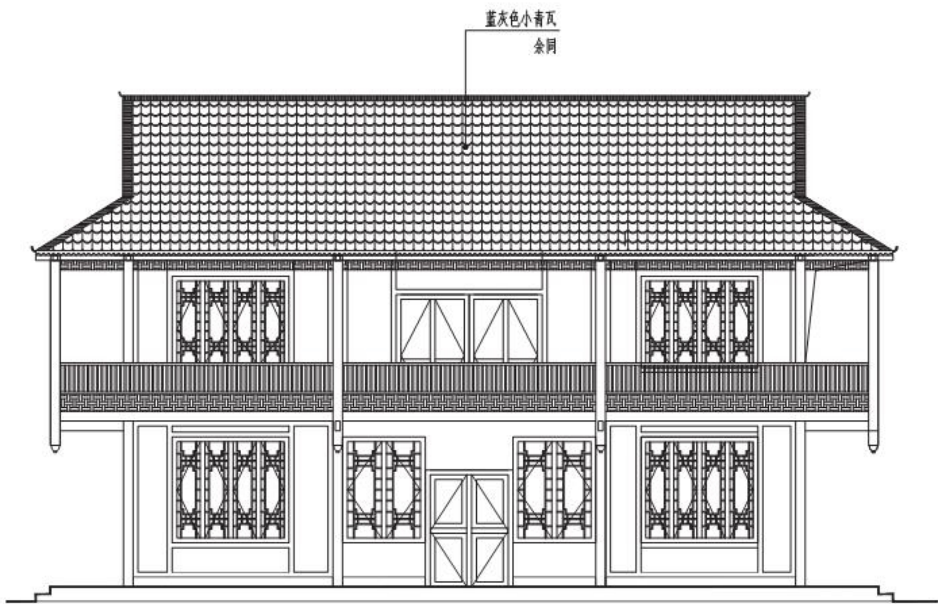
正立面图
