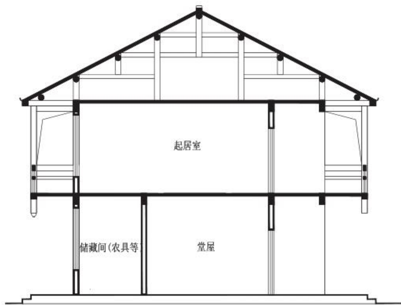
剖面图
