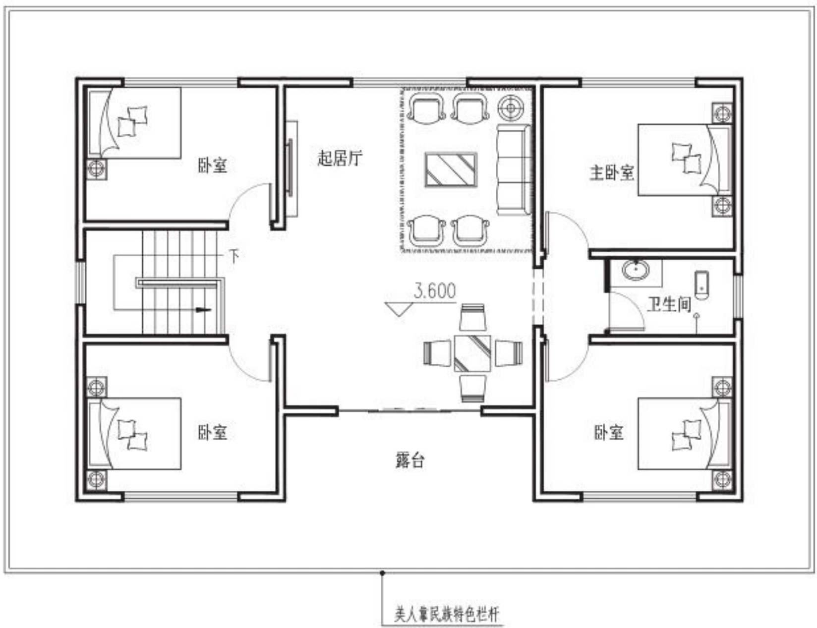
二层平面图
